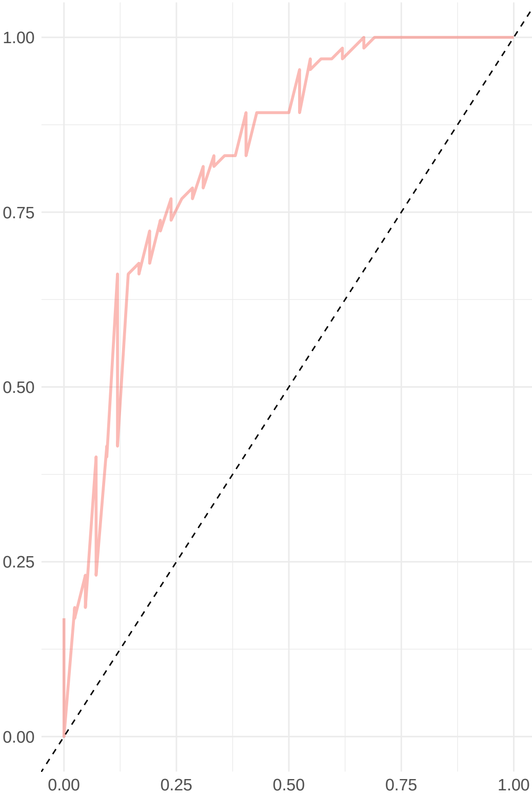
Backwards (AUC = 0.828)
