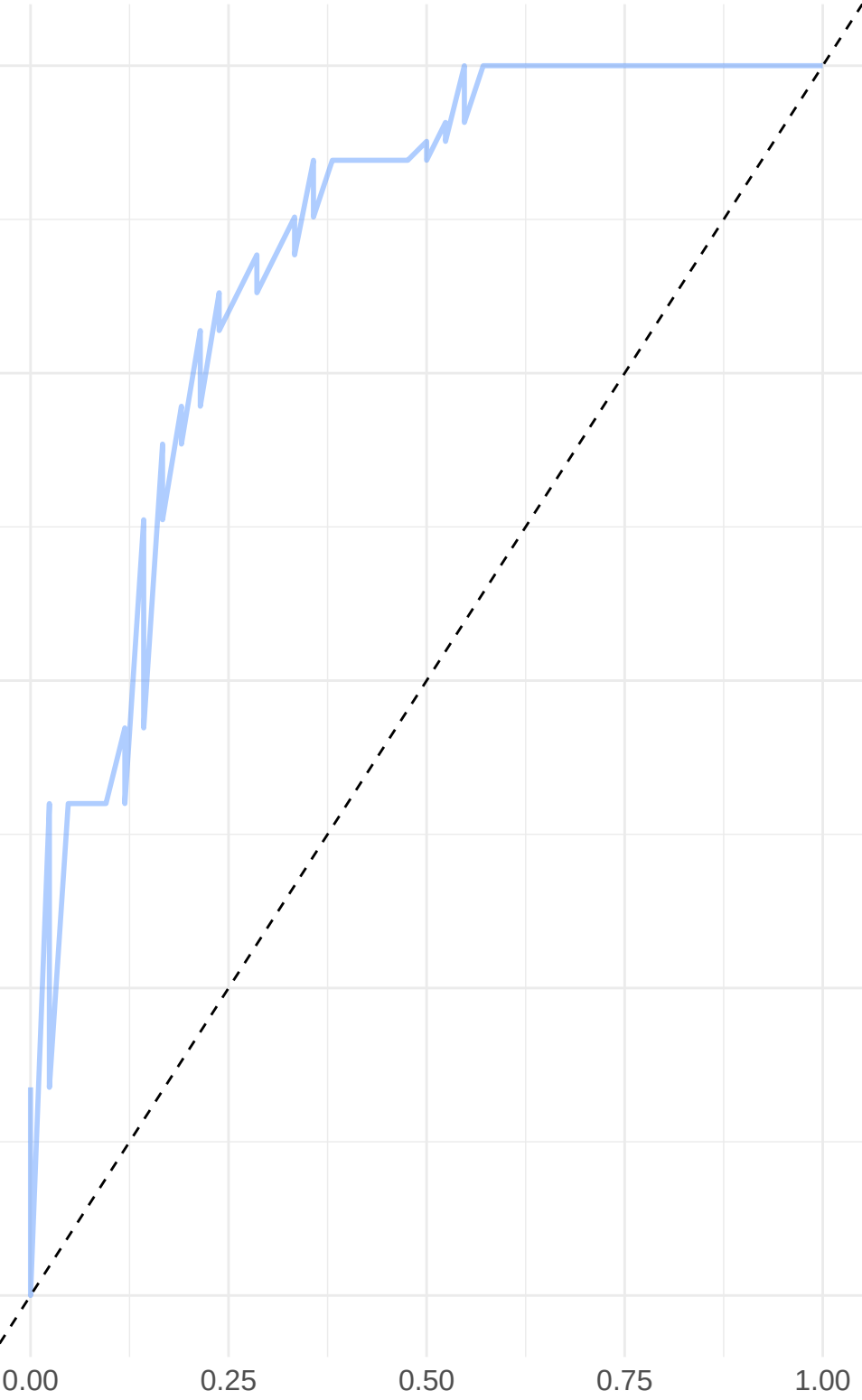
Forwards (AUC = 0.85)
